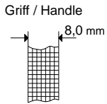
Barraquer 13cm / 5" Ohne Sperre / Without Catch M 1:1
