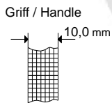
Kräftiger Koronar Nadelhalter Heavy Koronar Needle Holder 18cm / 7" Mit Sperre / With Catch M 1:1
